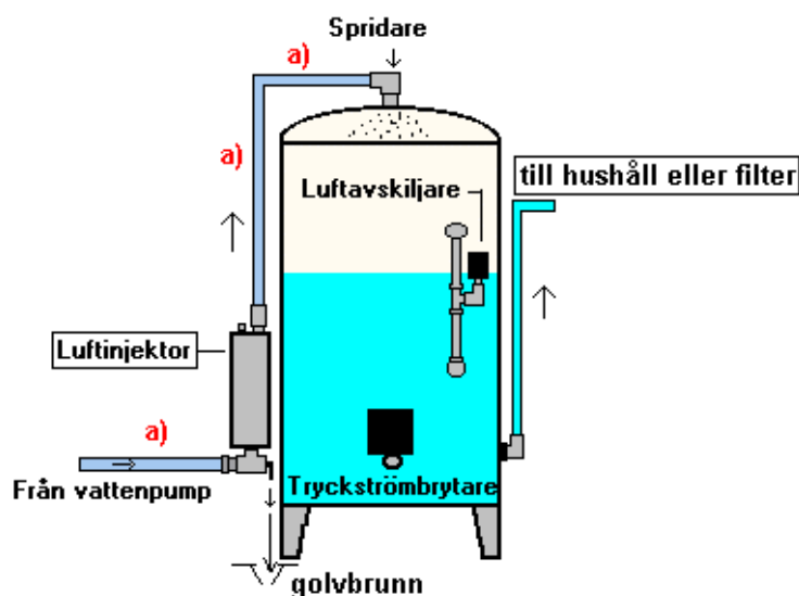
Denna bild visar enkel inkopplingskiss
